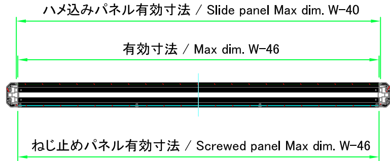
A-A ( 1 : 8 )
