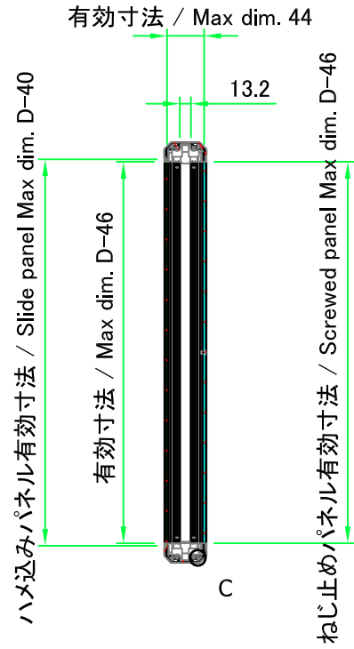
B-B ( 1 : 8 )
